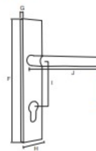
*R: Redonda
