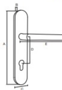
*R: Redonda
